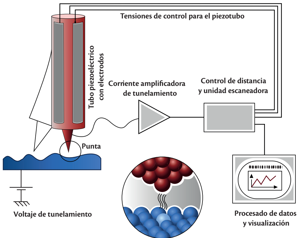
Figura 1. Esquema de funcionamiento de un microscopio de efecto túnel (STM). Crédito de la imagen: Área de Diseño Gráfico, Secretaría Técnica, IB-UNAM, modificado de A. Lusiardi (2014).
