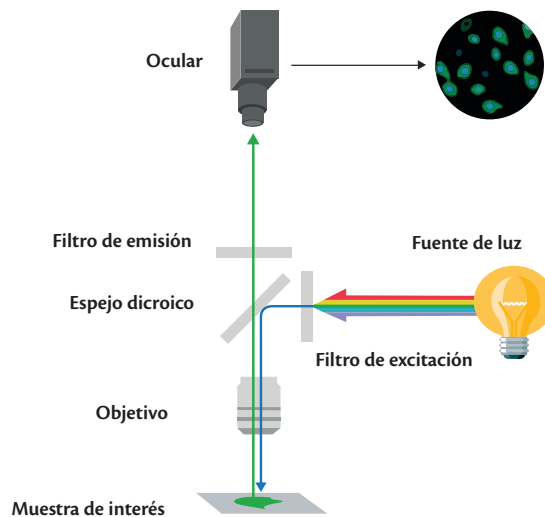
Figura 1. Representación esquemática del diseño de un microscopio de fluorescencia y micrografía. Crédito de la imagen: Área de Diseño Gráfico, Secretaría Técnica, IB-UNAM.
