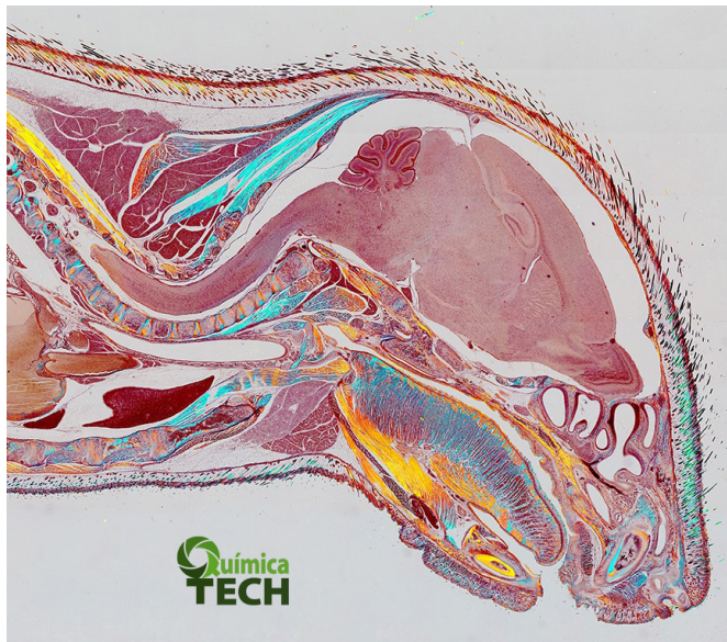
Figura 2. Corte de un feto de ratón sin teñir en donde los colores observados son el producto del estrés mecánico que hay en los tejidos y que pueden ser contrastados usando luz polarizada transmitida. Crédito de la imagen: Química Tech, S.A. de C.V.
