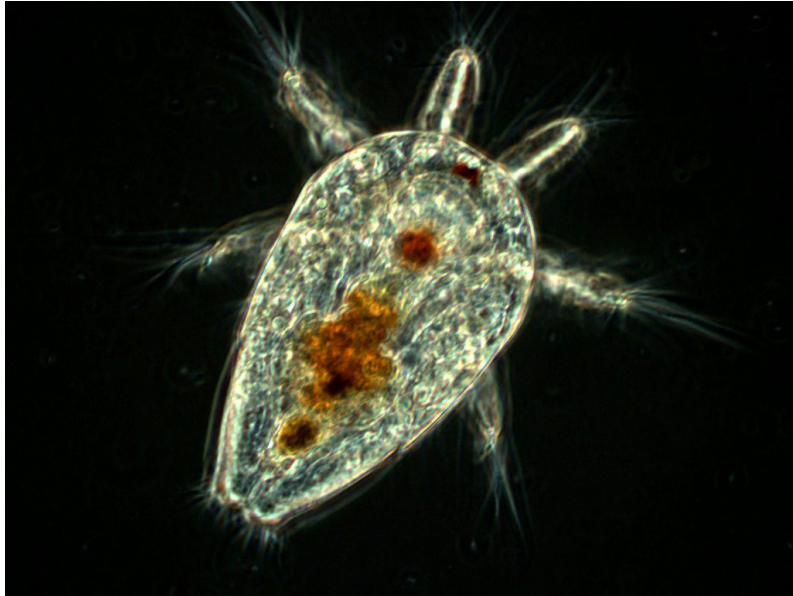
Figura 2. Copépodo visto por contraste de fases con 40x en muestra de agua de estanque. Crédito de la imagen: Gastón Contreras Jiménez.
