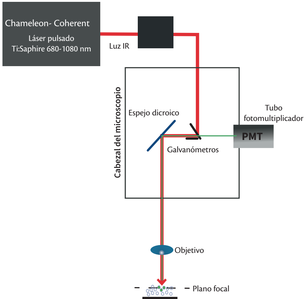
Figura 1. Esquema de componentes básicos de un microscopio de excitación de dos fotones. Se muestra: la fuente de luz (láser infrarrojo pulsado), que va de 680-1 080 nm; el modulador acusto-óptico, que atenúa el poder del láser; el espejo dicroico, que deja pasar la luz infrarroja y refleja la luz emitida; el tubo fotomultiplicador (PMT), y el objetivo. Crédito de la imagen: Yazmín Ramiro Cortés, modificada por el Área de Diseño Gráfico, Secretaría Técnica, IB-UNAM.
