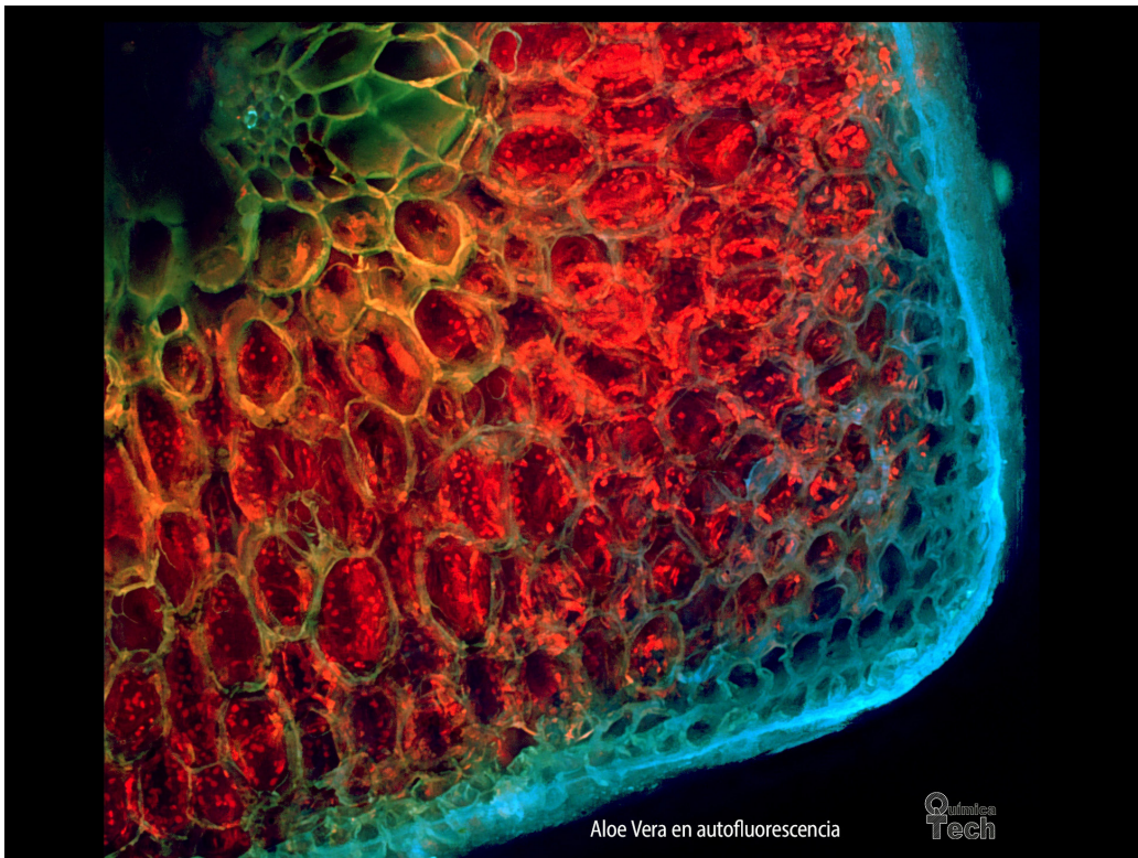
Figura 3. Corte transversal de una hoja de Aloe vera en fluorescencia (esta imagen ganó el premio People award del concurso de la Microscopy Society of America en el 2020). Crédito de la imagen: Química Tech S.A. de C.V.
